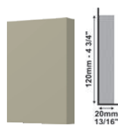
Sócalo 178 Cinza Glacial PLinth Glacial Gray Zócalin Gris Glacial 80 x 120 x 20mm 3 1/8" x 4 3/4" x 13/16" Cód. | Code - 21387
