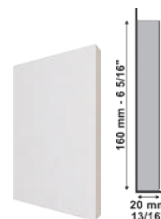
Sócalo 187 | Plinh | Zócalin 110 x 160 x 20mm 4 3/8" x 6 5/16" x 13/16" Cód. | Code - 27377
