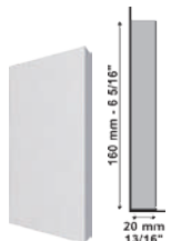
Sócalo 186 | Plinh | Zócalin 80 x 160 x 20mm 3 1/8" x 6 5/16" x 13/16" Cód. | Code - 27376
