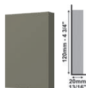
Sócalo 178 Cinza Titanium PLinth Titanium Gray Zócalin Gris Titanio 80 x 120 x 20mm 3 1/8" x 4 3/4" x 13/16" Cód. | Code - 21388
