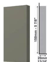
Sócalo 183 Cinza Titanium PLinth Titanium Gray Zócalin Gris Titanio 70 x 150 x 20mm 2 3/4" x 5 7/8" x 13/16" Cód. | Code - 21390
