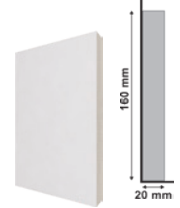
Sócalo 187 Plinth Block | Zócalin 110 x 160 x 20mm Cód. | Code - 25362
