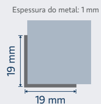
Cantoneira Metálica Alumínio Anodizado Anodized Aluminum Metallic Angle Cantonera Metalica de Aluminio Anodizado Cód. | Code - 21482
