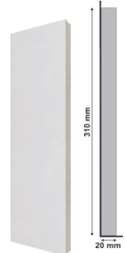
Sócalo 188 Plinth Block | Zócalin 110 x 310 x 20mm Cód. | Code - 25363
