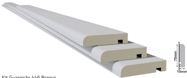
Kit Guarnição 446 Branco White Architrave Pro Pack 446 | Kit Contramarco 446 Branco Cód | Code - 20335
