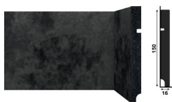
3496 RP OXI Preto OXI Black Skirting Board | Zócalo OXI Negro Cód. | Code - 28585
