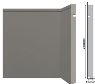
520 RP/Cinza Titanium Titanium Gray Skirting Board Zócalo Gris Titanio
