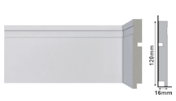
493 RP/BR White Skirting Board | Zócalo Blanco Cód. | Code - 24574
