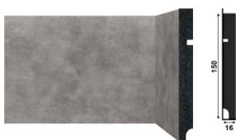
3496 RP OXI Prata OXI Silver Skirting Board | Zócalo OXI Plata Cód. | Code - 28586
